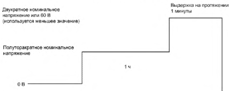
Рисунок 2 — Цикл испытания на воздействие повышенных электрических напряжений
